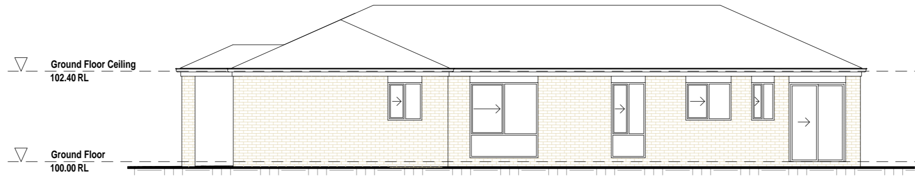
1 Elevation A 1 : 100
